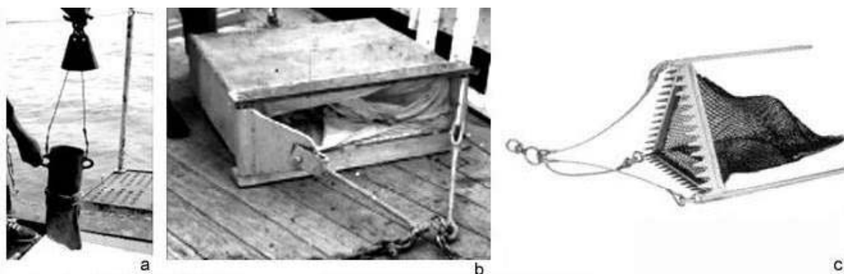
Figura 1 - Dragas: a - Draga Gibbs; b - Draga retangular; c - Draga de rochas.
