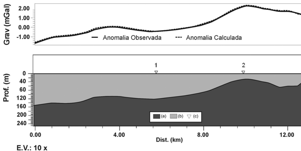
Figura 15 – Perfil 1: anomalias gravimétricas (observada – linha cheia; calculada – linha tracejada) e o modelo geológico. (a) embasamento indiferenciado ( \rho = 2,8 \text{ g/cm}^3 ); (b) sedimentos indiferenciados ( \rho = 2,0 \text{ g/cm}^3 ); (c) pontos de referência.
