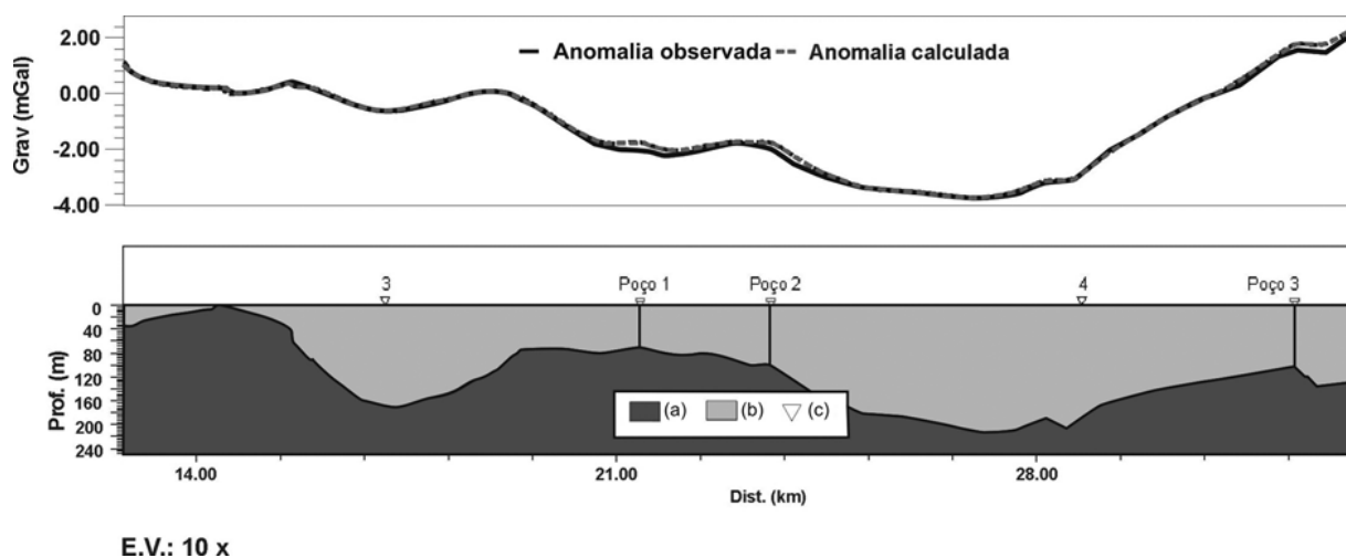
Figura 16 – Perfil 2a: anomalias gravimétricas (observada – linha cheia; calculada – linha tracejada) e o modelo geológico. (a) embasamento indiferenciado ( \rho = 2,8 \text{ g/cm}^3 ); (b) sedimentos indiferenciados ( \rho = 2,0 \text{ g/cm}^3 ); (c) pontos de referência.
