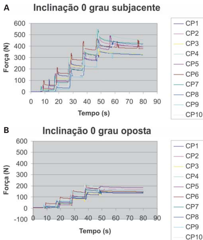
Gráfico 1 – Demonstração de valores médios da força máxima de compressão axial posições do virtual foco de fratura. A) Cortical subjacente à placa; B) Cortical oposta à placa.
