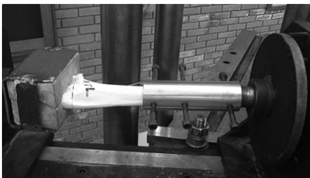
Fig. 5 Mecanismo para aplicação das cargas torcionais.
