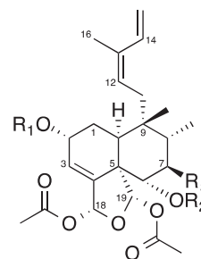
1 R 1 = n -C 3 H 7 CO; R 2 =R 3 =H 2 R 1 =CH 3 ; R 2 =CH 3 CO; R 3 = n -C 3 H 7 -COO
