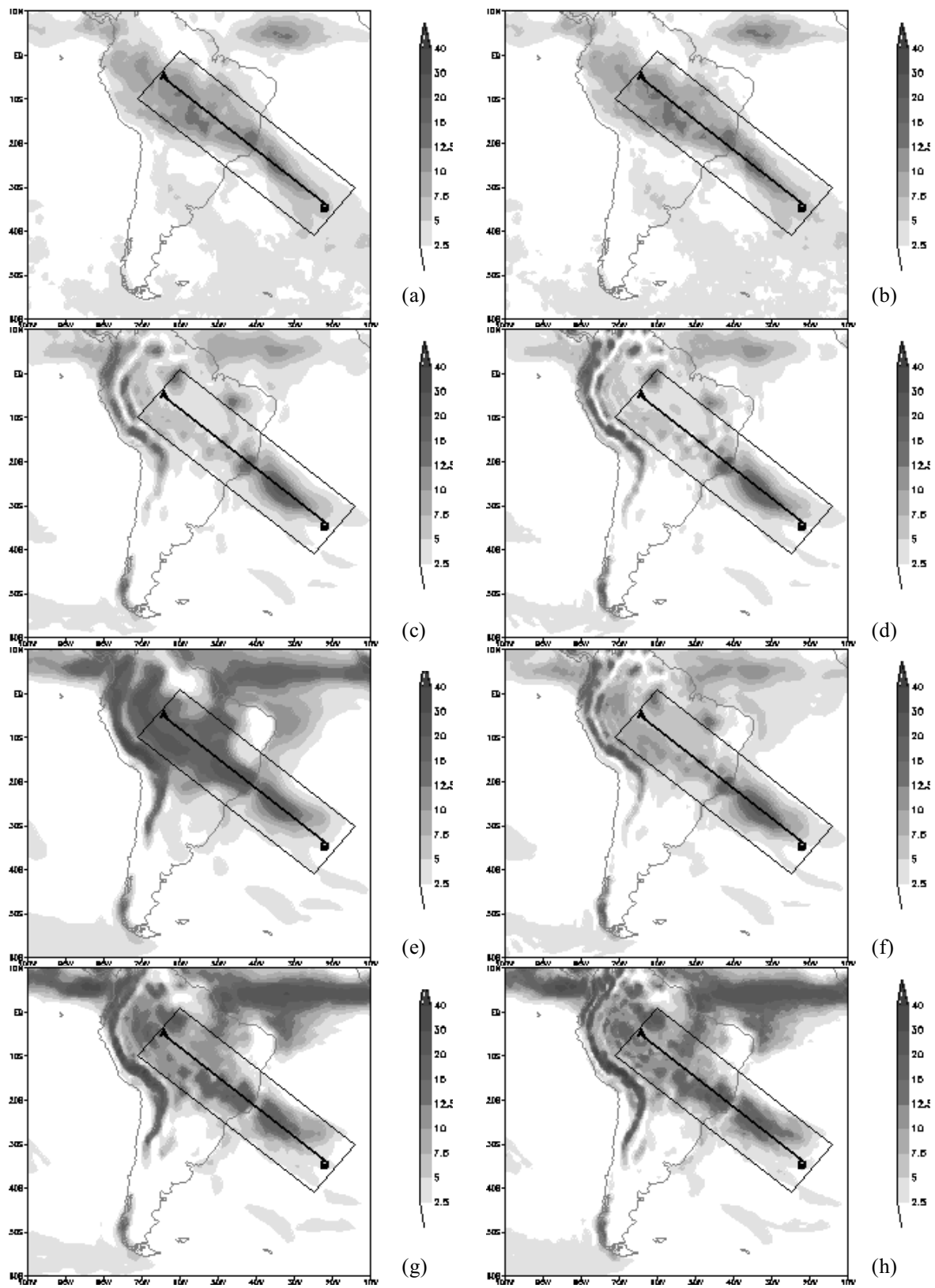
Figura 6 – Precipitação Total (mm/dia), para o composto de ZCAS: (a) e (b) dados GPCP, (c)-(h) MCGA-CPTEC – KUO, RAS e GRELL respectivamente, para as resoluções T126L28 (a esquerda) e T170L42 (a direita).
