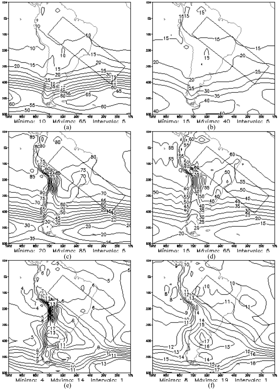
Figura 3 – Energia Total (%), MCGA-CPTEC – KUO, média das previsões de 24h, T126L28 (a esquerda) e T170L42 (a direita): (a) e (b) modos verticais 1 a 3; (c) e (d) modos verticais 4 a 7; e (e) e (f) modos verticais 8 a 12 (8 a 14, para T170L42).
