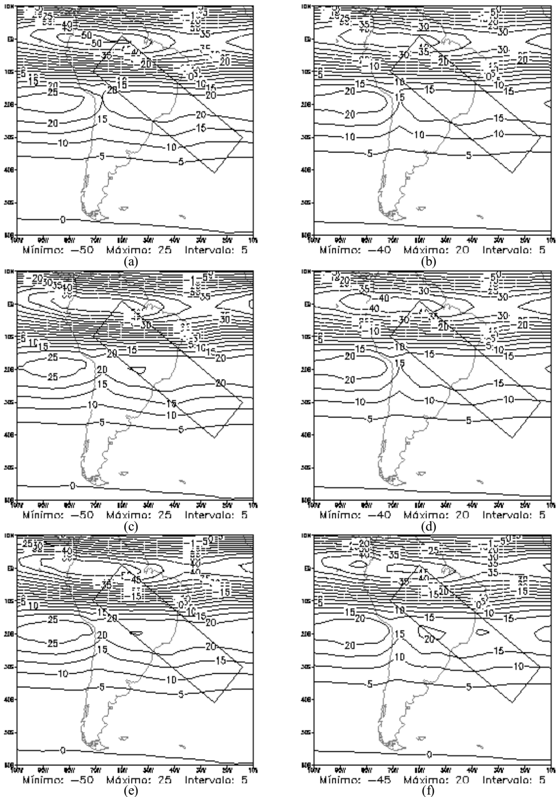
Figura 12 – Energia Total (%) das interações entre os modos Rossby e Kelvin, para os modos verticais 4 a 7, média das previsões de 24h, MCGA-CPTec - T126L28 (a esquerda) e T170L42 (a direita): (a) e (b) KUO; (c) e (d) RAS; (e) e (f) GRELL.
