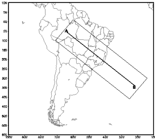
Figura 2 – Região média de atuação do composto de ZCAS, definida para a partição modal vertical de energia sobre a América do Sul.
