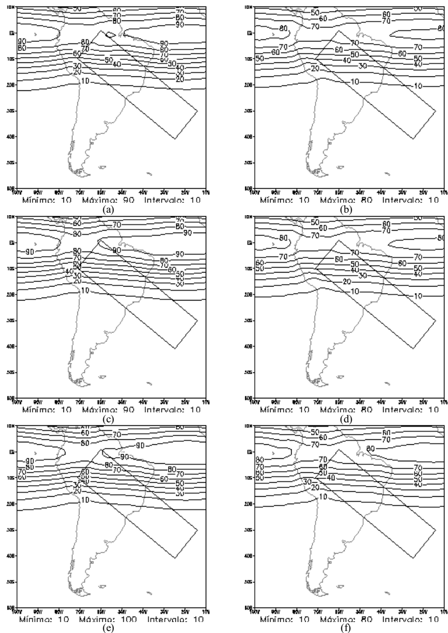
Figura 10 – Energia Total (%) do modo horizontal Kelvin para os modos verticais 4 a 7, média das previsões de 24h, MCGA-CPTEC - T126L28 (a esquerda) e T170L42 (a direita): (a) e (b) KUO; (c) e (d) RAS; (e) e (f) GRELL.
