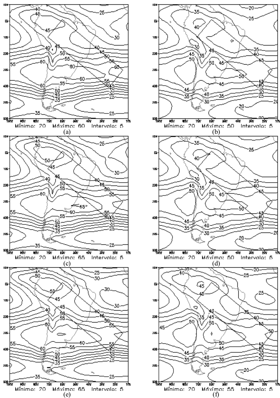
Figura 9 – Energia Total (%) do modo horizontal Rossby para os modos verticais 4 a 7, média das previsões de 24h, MCGA-CPTEC - T126L28 (a esquerda) e T170L42 (a direita): (a) e (b) Kuo; (c) e (d) RAS; (e) e (f) GRELL.
