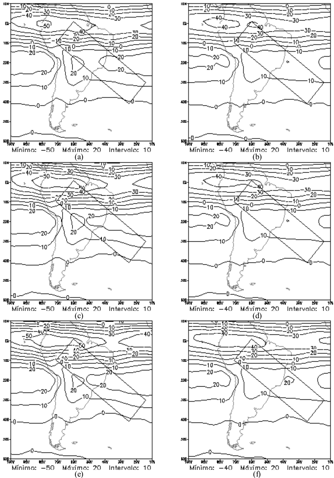
Figura 11 – Energia Total (%) da soma de todas as interações - Resíduo, para os modos verticais 4 a 7, média das previsões de 24h, MCGA-CPTEC - T126L28 (a esquerda) e T170L42 (a direita): (a) e (b) KUO; (c) e (d) RAS; (e) e (f) GRELL.
