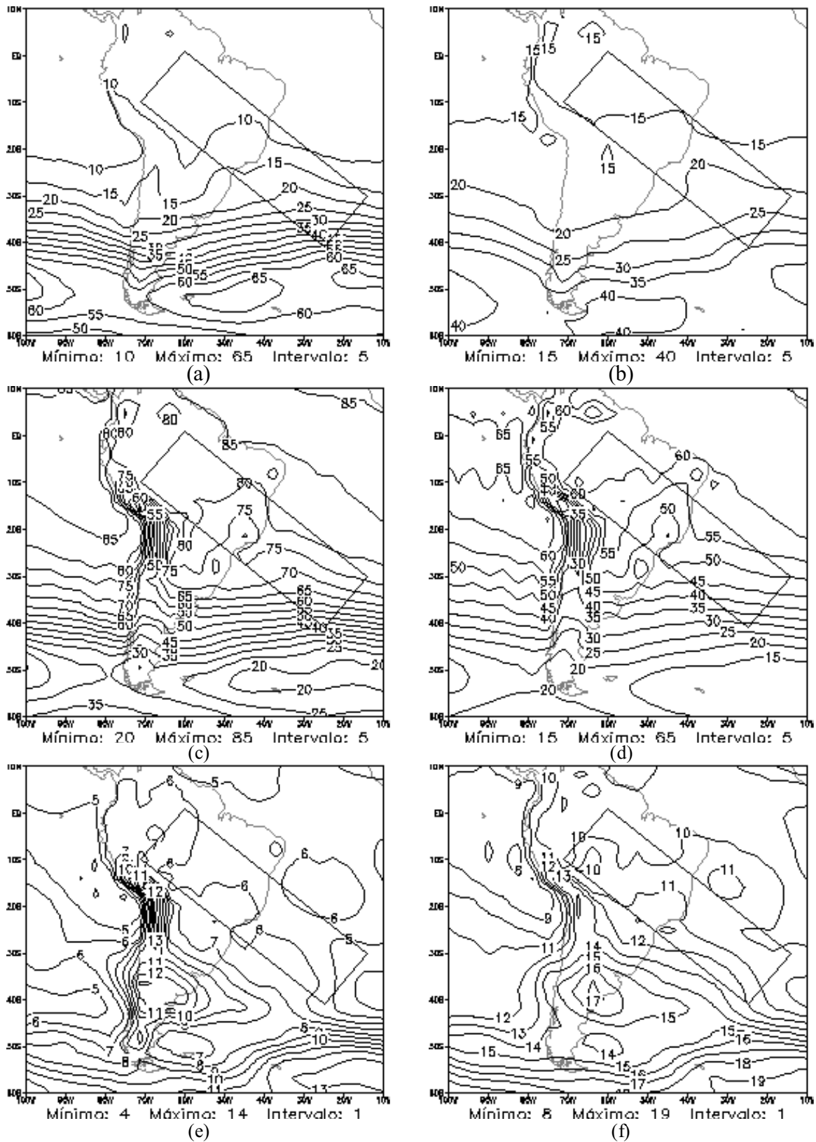
Figura 4 – Energia Total (%), MCGA-CPTEC – RAS, média das previsões de 24h, T126L28 (a esquerda) e T170L42 (a direita): (a) e (b) modos verticais 1 a 3; (c) e (d) modos verticais 4 a 7; e (e) e (f) modos verticais 8 a 12 (8 a 14, para T170L42).
