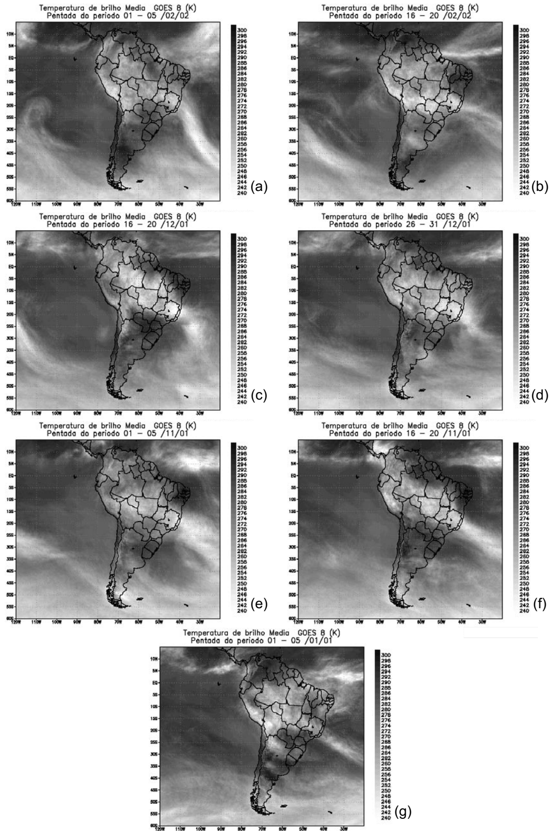
Figura 1 – Temperatura de Brilho Média para pêntadas referentes aos episódios de ZCAS selecionados. FONTE: Metop/CPTEC/INPE.
