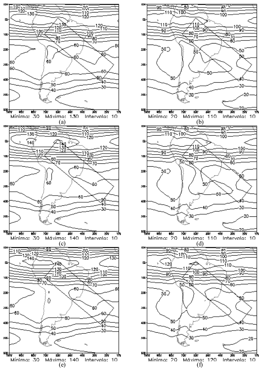
Figura 8 – Energia Total (%) do modo horizontal Soma para os modos verticais 4 a 7, média das previsões de 24h, MCGA-CPTEC - T126L28 (a esquerda) e T170L42 (a direita): (a) e (b) Kuo; (c) e (d) RAS; (e) e (f) Grell.
