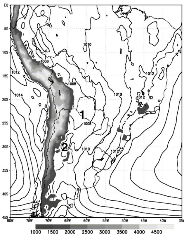
Figura 1 - Campo médio de pressão ao nível médio do mar (hPa) para os meses de verão (dezembro a fevereiro), construído a partir das reanálises do modelo regional Eta/CPTEC para o período 2000-2004. Os tons de cinza indicam elevações acima do nível médio do mar (m). 1: BCH, 2: BNOA
