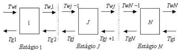
Figura 5: Esquema do modelo do trocador de calor com N estágios de troca térmica.
