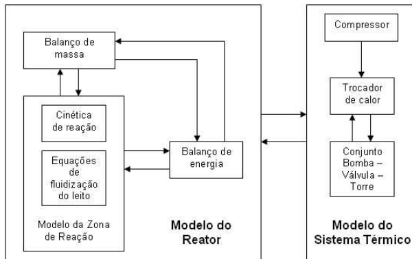
Figura 2: Esquema do modelo do processo UNIPOL®
