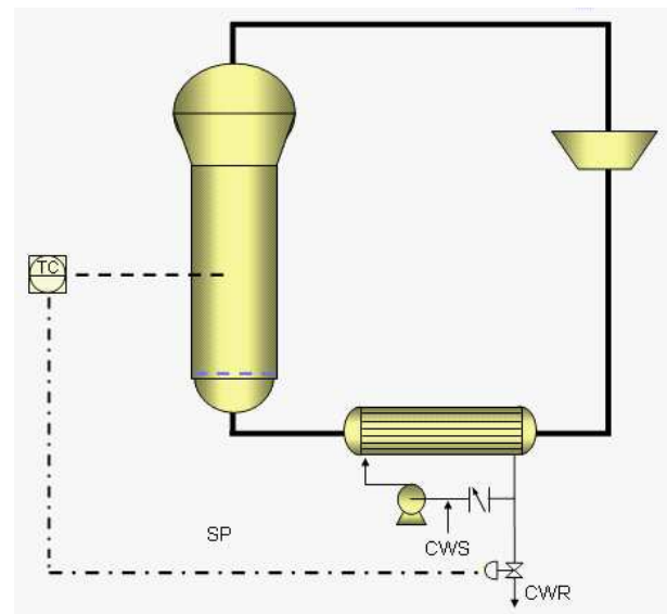
Figura 18: Esquema do controlador PID para temperatura do reator.
