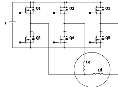
Figura 2: Inversor de tensão bifásico com três braços.
