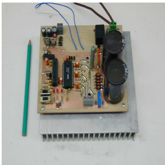
Figura 6: Foto do protótipo implementado.
