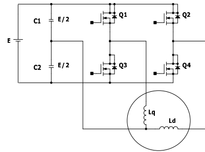
Figura 1: Inversor de tensão bifásico H-bridge.
