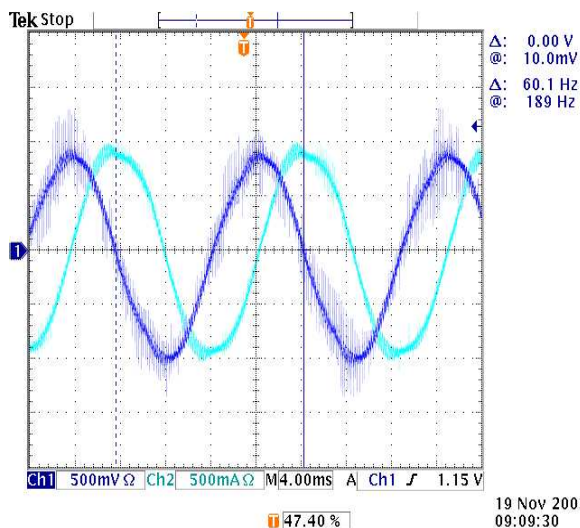
Figura 7: Correntes de estator com frequência de 60Hz.
