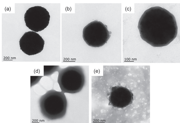
Figure 2. TEM images of (a) \text{Fe}_3\text{O}_4 ; (b) \text{Fe}_3\text{O}_4@SiO_2 ; (c) \text{Fe}_3\text{O}_4@MPS ; (d) MMIP and (e) MMIC.
