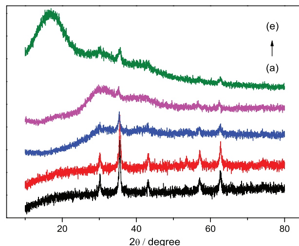
Figure 4. XRD images of (a) \text{Fe}_3\text{O}_4 ; (b) \text{Fe}_3\text{O}_4@SiO_2 ; (c) \text{Fe}_3\text{O}_4@MPS ; (d) MMIP and (e) MMIC.
