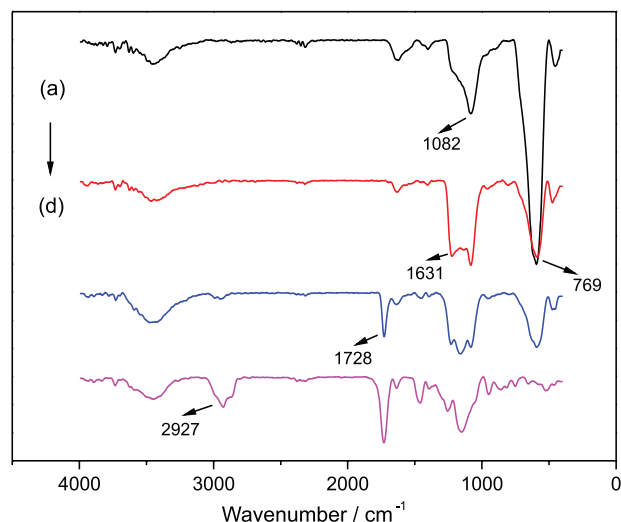
Figure 3. FTIR images of (a) \text{Fe}_3\text{O}_4@SiO_2 ; (b) \text{Fe}_3\text{O}_4@MPS ; (c) MMIP and (d) MMIC.
