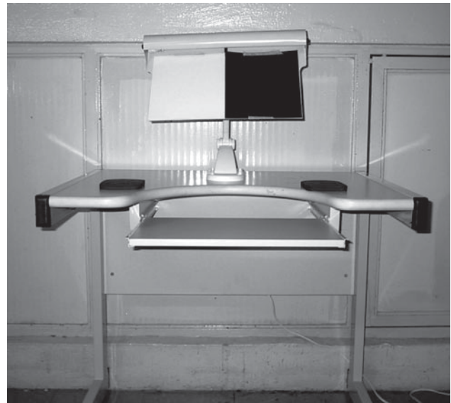
Figura 15: Vista geral do protótipo III.
