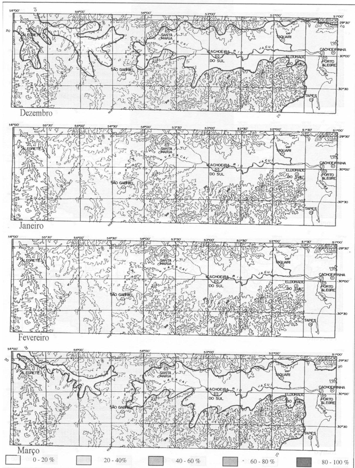
Figura 5 - Probabilidade da ocorrência de dez ou mais dias com temperatura mínima igual ou inferior a 15°C nos meses de dezembro, janeiro, fevereiro e março no Região Climática da Depressão Central, Estado do Rio Grande do Sul.
