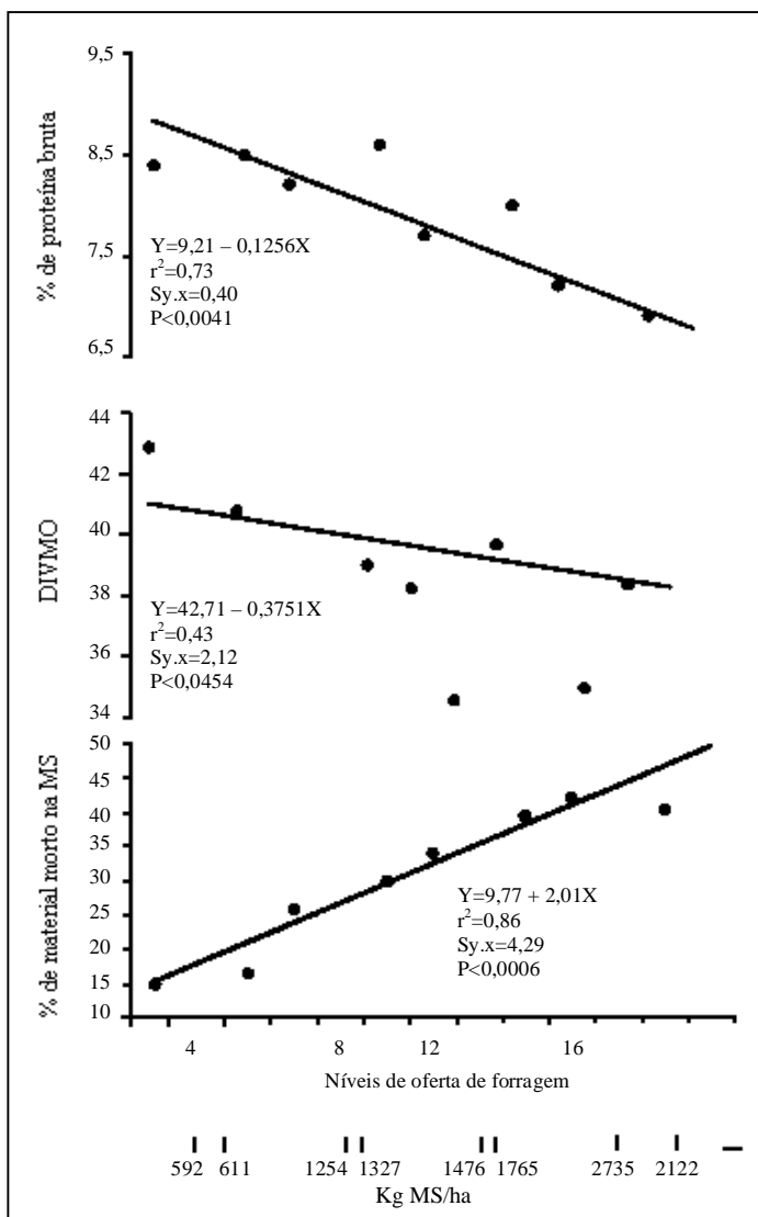
Figura 2 – Porcentagem de proteína bruta média, digestibilidade da matéria orgânica % e porcentagem de material morto do campo nativo submetido a níveis de oferta de forragem. EEA, UFRGS, Eldorado do Sul.
