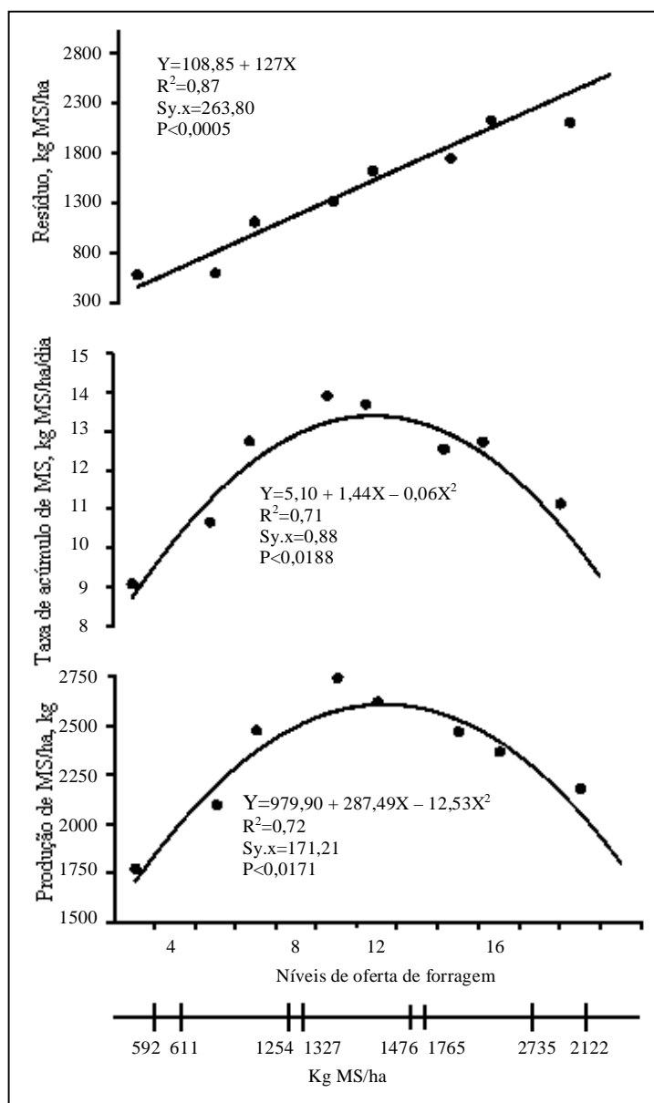
Figura 1 – Resíduos kg MS/ha, taxa de acumulação de MS (kg MS/ha/dia) e produção de MS/ha (kg) do campo nativo submetido a níveis de oferta de forragem. EEA,UFRGS, Eldorado do Sul.
