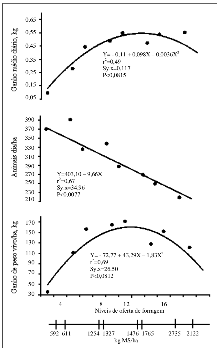
Figura 3 - Ganho médio diário (kg), animais dia/ha (nº) e ganho de peso vivo/ha (kg) no campo nativo submetido a níveis de oferta de forragem. EEA, UFRGS, Eldorado do Sul.
