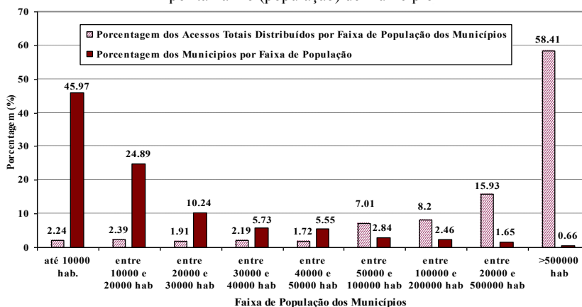
Gráfico 5 Distribuição das porcentagens de acesso de Banda Larga por tamanho (população) de município
