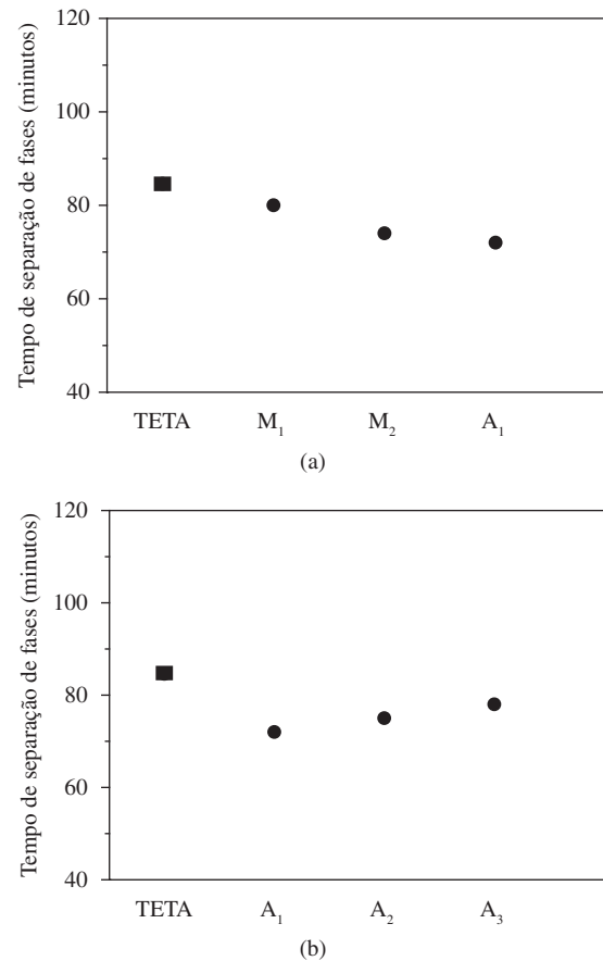
Figura 4. Tempo de gelificação para o adesivo puro (TETA) e tempo de separação de fases dos adesivos com 10 phr de copolímero acrílico. a) com diferente massa molecular; M_1 ( \overline{M}_n = 8,74 \times 10^3 ); M_2 ( \overline{M}_n = 3,40 \times 10^3 ); A_1 ( \overline{M}_n = 1,19 \times 10^4 ); e b) com diferente concentração de grupos carboxílicos; A_1 ( 0,00 \text{ mmol g}^{-1} ); A_2 ( 8,30 \times 10^{-2} \text{ mmol g}^{-1} ); e A_3 ( 2,90 \times 10^{-1} \text{ mmol g}^{-1} ).
