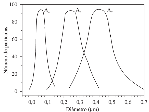
Figura 7. Influência da concentração de grupos carboxílicos na curva de distribuição de tamanhos para os adesivos com 10 phr de copolímero acrílico; A 2 (8,30 × 10 -2 mmol g -1 ); A 3 (2,90 × 10 -1 mmol g -1 ); e A 4 (4,06 × 10 -1 mmol g -1 ) após o programa de cura de duas etapas.
