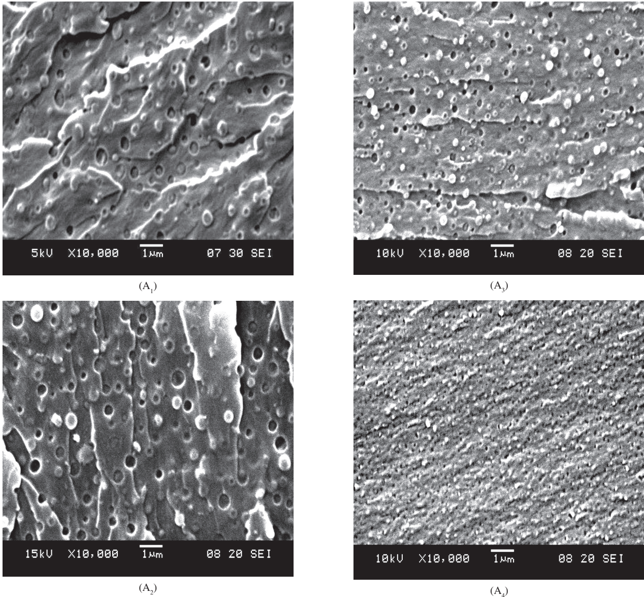
Figura 6. Micrografias eletrônicas (SEM) da superfície de fratura dos adesivos com diferente concentração de grupos carboxílicos; A 1 (0,00 mmol g -1 ); A 2 (8,30 × 10 -2 mmol g -1 ); A 3 (2,90 × 10 -1 mmol g -1 ); e A 4 (4,06 × 10 -1 mmol g -1 ) após o programa de cura de duas etapas.
