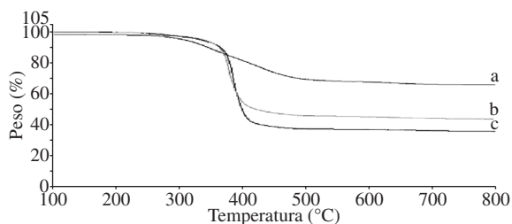
Figura 6. Curvas de termogravimetria para: a) viscolgel B8; b) mistura física de viscolgel B8-PEG; e c) reação viscolgel B8-PEG.
