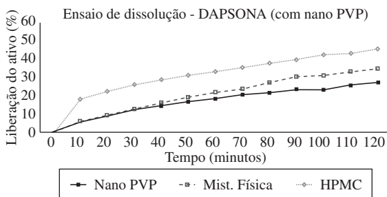
Figura 10. Perfil de dissolução em SGS do nanocompósito viscogel B8-PVP K-30, da mistura física e HPMC.
