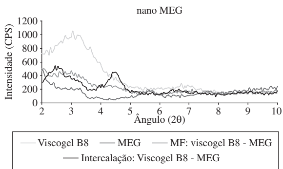
Figura 1. Difratograma da intercalação viscogel B8-MEG.
