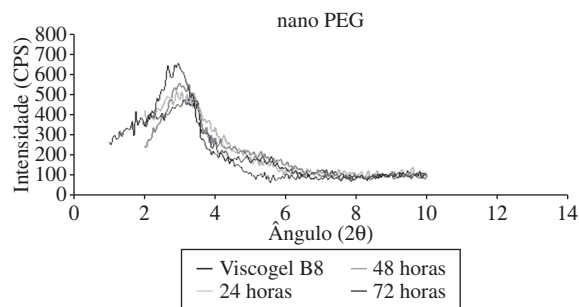
Figura 4. Difratograma das reações viscogel B8-PEG sob refluxo.
