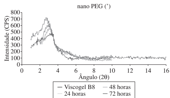
Figura 5. Difratograma das reações viscogel B8-PEG a temperatura ambiente.
