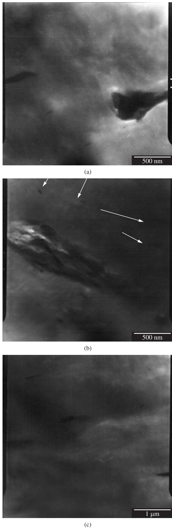
Figura 5. Micrografias dos nanocompósitos com 3% em massa de argila organofílica modificada com Cetremide® (ACT): a) PE/ACT; b) PE-g-MA/ACT; e c) PE/PE-g-MA/ACT [38] .
