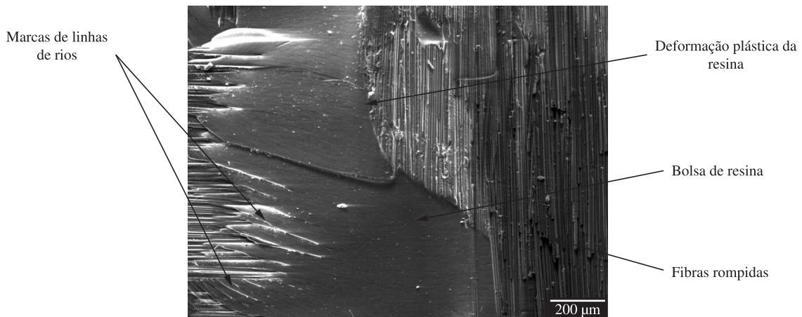
Figura 9. Superfície de fratura do laminado carbono/epóxi (região A). Detalhe de bolsa de resina (região inferior).
