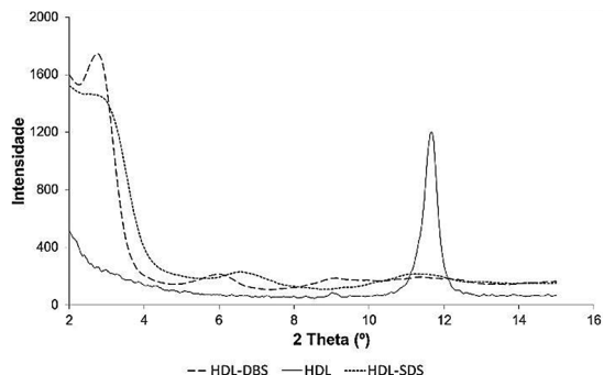
Figura 4. Difratoograma de raios-X para baixos ângulos para HDL, HDL-DBS e HDL-SDS.
