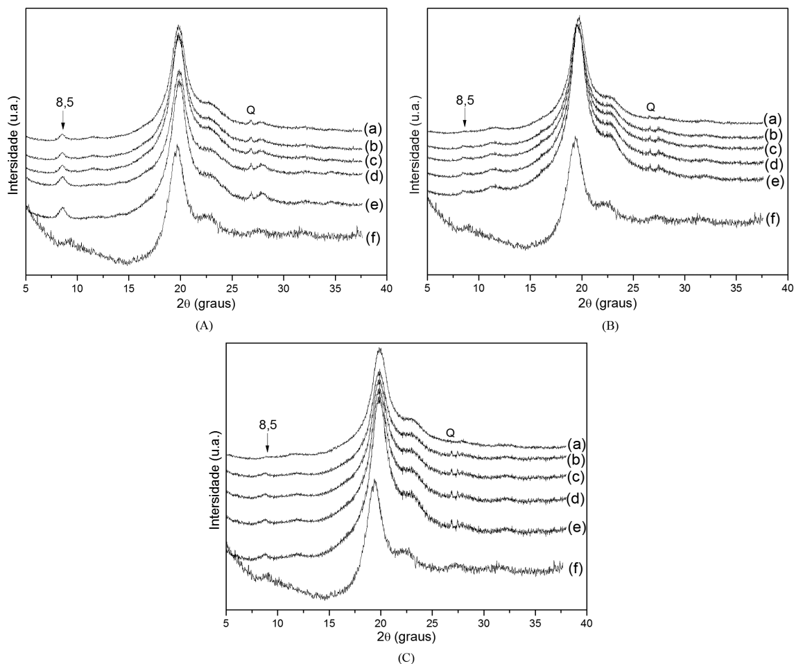
Figura 6. Difratogramas de raios x dos filmes de PVA contendo o argilomineral (A), e dos materiais híbridos PGS/AM (B) e PGS/VC (C) com diferente percentagem em relação a massa do PVA: (a) 0%; (b) 2%; (c) 3%; (d) 5%; (e) 8%; (f) 0%. Todas as análises foram realizadas na parte superior dos filmes. Contaminante: (Q = quartzo).
