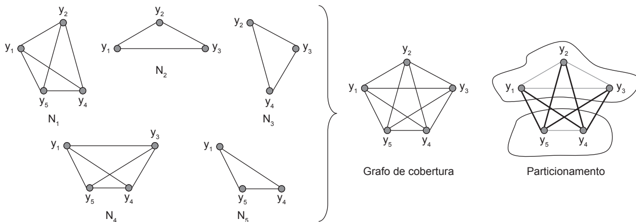
Figura 3. Exemplo de um grafo de cobertura.
