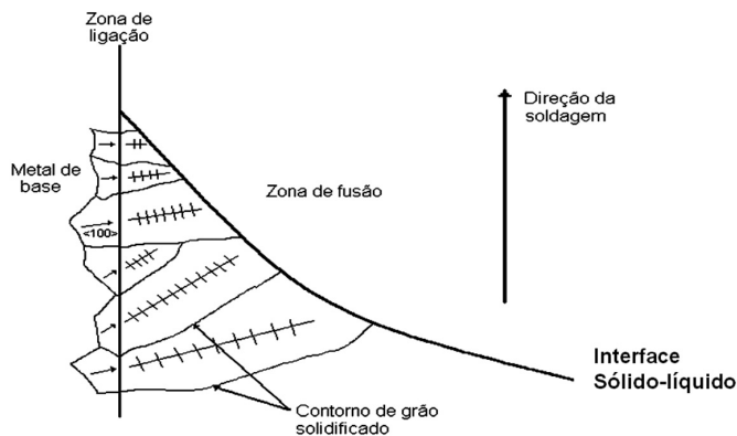
Figura 4. Representação esquemática do crescimento epitaxial e crescimento competitivo dos grãos da ZF [13].
