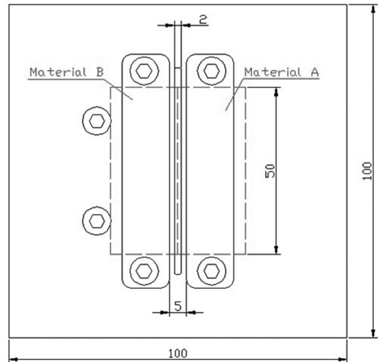
Figura 6. Dispositivo desenvolvido para fixação e soldagem dos metais de base.
