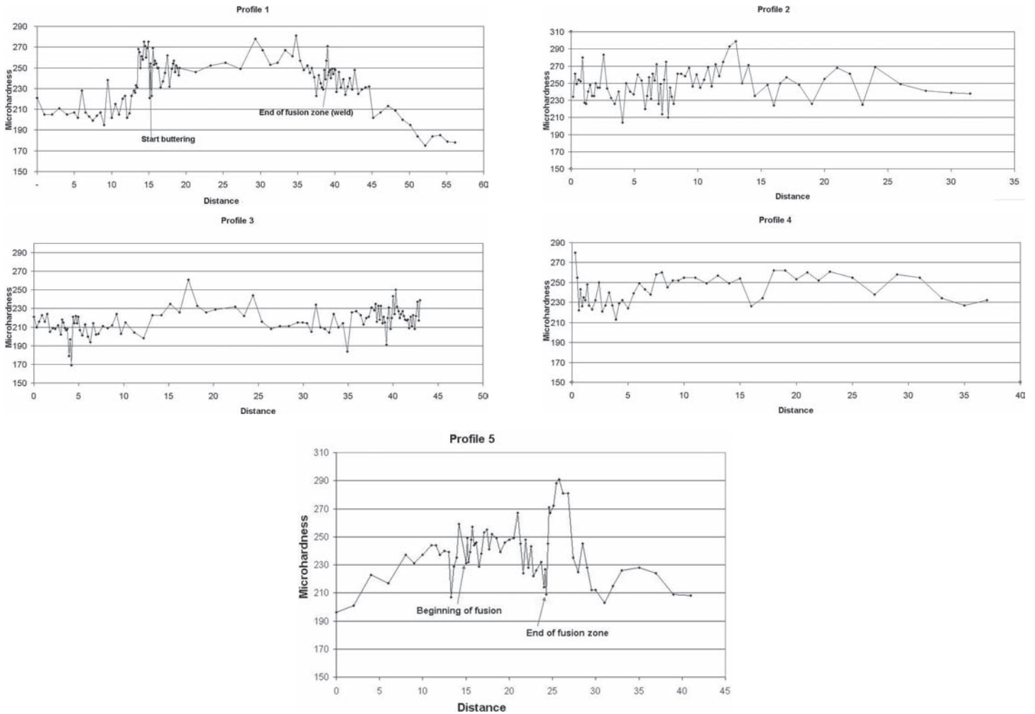
Figura 15 – Perfis de microdureza da junta dissimilar.
