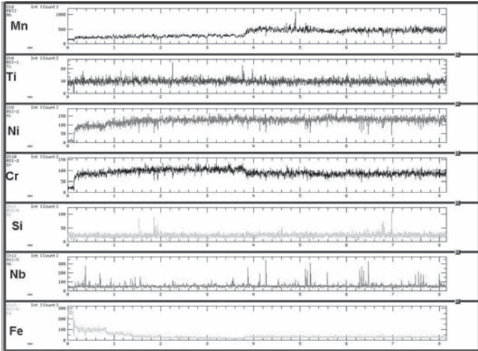
Figura 13 – Perfil da composição dos elementos Mn, Ti, Ni, Cr, Si, Nb e Fe feito no metal base ASTM A-508 G3 em direção a zona fundida da liga 182.
