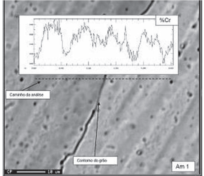
Figura 14 - Microfotografia obtida no MEV e análise por EDS mostrando a variação intradendrítica do teor de cromo na liga 182.
