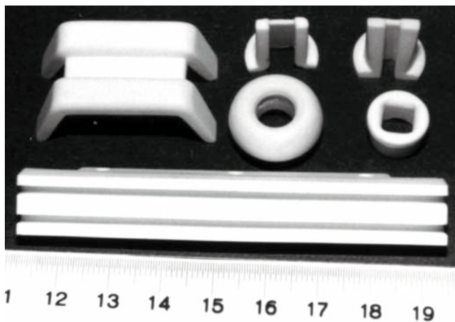
Figura 4: Guia-fios sinterizados com parede fina.
