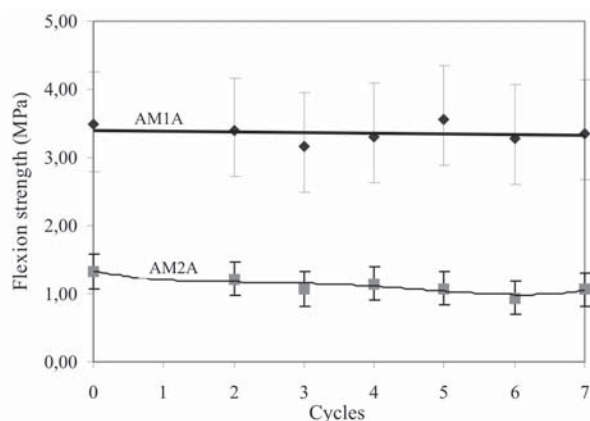
Figure 8: Average flexion strength of the AM1 and AM2 mortars subjected to wetting and drying cyclic period after 28-day aging time. [Figura 8: Resistência à flexão média das argamassas AM1 e AM2 submetidas a períodos cíclicos de molhagem e secagem após 28 dias de cura.]
