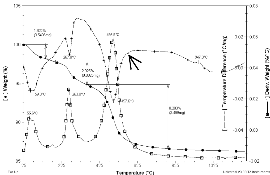
Figura 3: Curvas de análise térmica (ATD/TG/DTG) da “fração total”, < 840 \mu\text{m} . [Figure 3: Thermal analysis curves (DTA/TG/DTG) of the “total fraction”, < 840 \mu\text{m} .]
