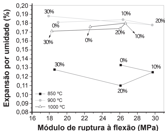
Figura 5: EPU versus módulo de ruptura à flexão de corpos cerâmicos autoclavados contendo adições de 0, 10, 20 e 30% de quartzo [12].
