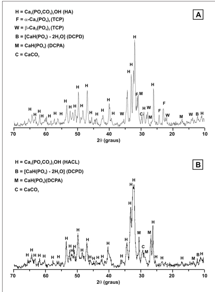
Figura 1 - Difractogramas dos pós de HA (a) e HA. CL (b).
