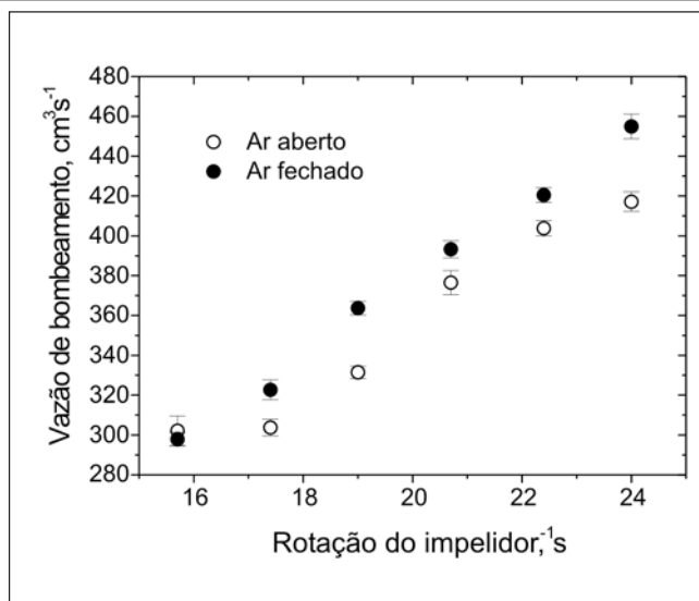
Figura 6 - Vazão de bombeamento ( Q_b ) versus rotação do impelidor.
