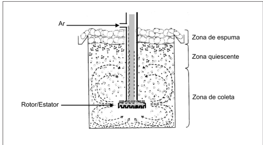
Figura 1 - Padrões de fluxo numa célula de flotação.
