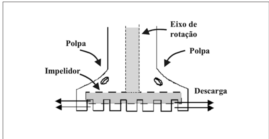
Figura 2 - Descarga de fluido na região rotor/estator.
