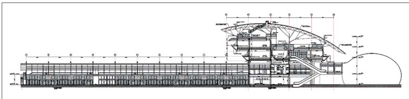
Figura 2 - Corte transversal do prédio central.
