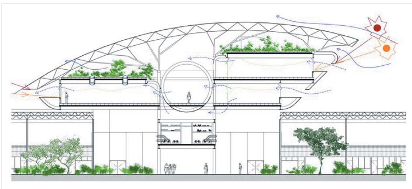
Figura 3 - Estruturas metálicas de coberturas e envoltórias.
