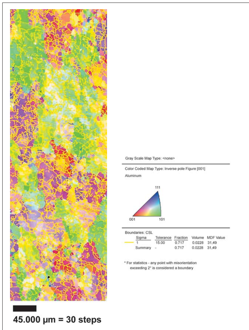
Figura 8 - Mapeamento de contornos CSL da amostra caster 1/2 de espessura, direção de laminação paralela à direção vertical.
