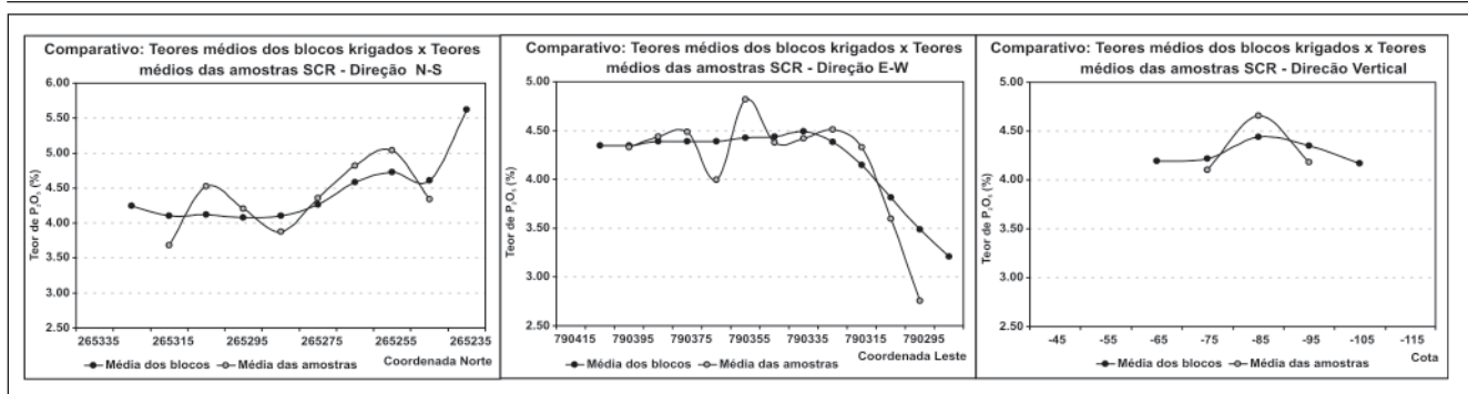
Figura 8 - Verificação dos resultados da krigagem de blocos com as amostras SCR.
