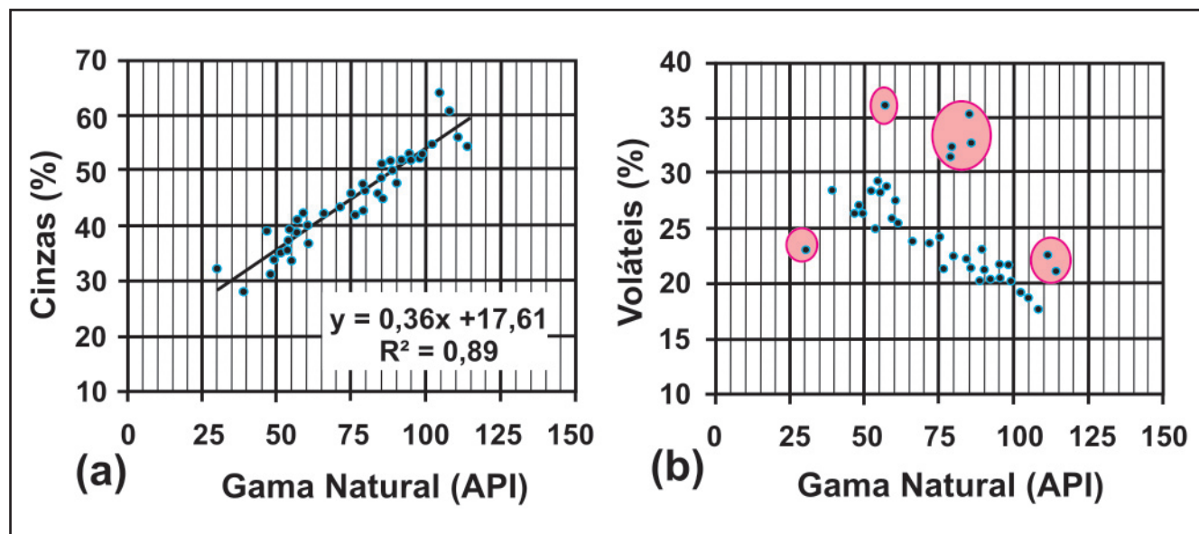
Figura 3 - (a) Modelo linear proposto para previsão do teor de cinzas (%) a partir do gama natural. (b) Gráfico de dispersão entre voláteis (%) e gama natural. Pontos circulado correspondem às amostras erráticas, apresentando, em sua maioria, voláteis acima de 30%.
