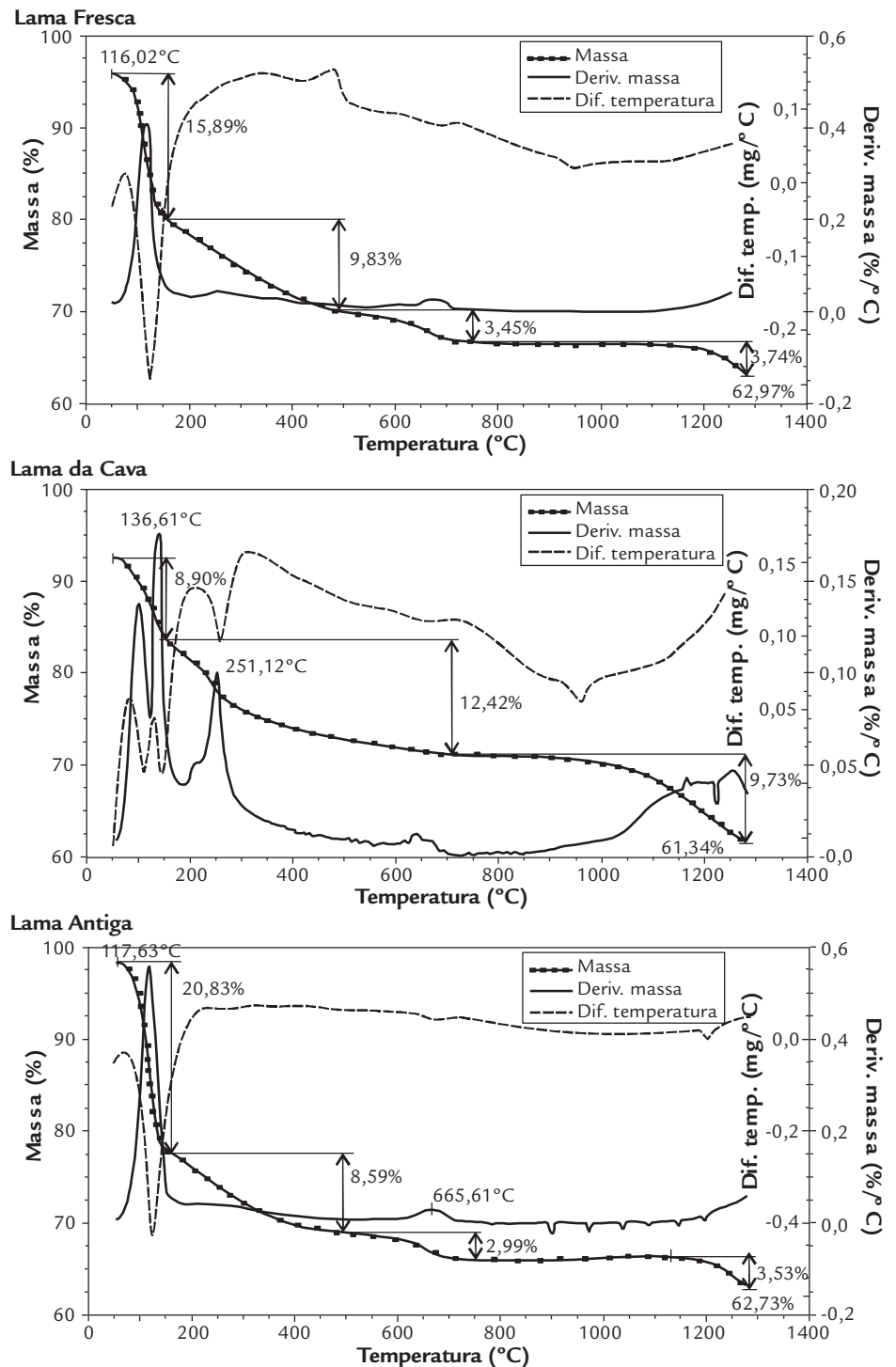
Figura 1 Diagrama TGA-DTA obtido para as amostras das Lamas Fresca, da Cava e Antiga.
