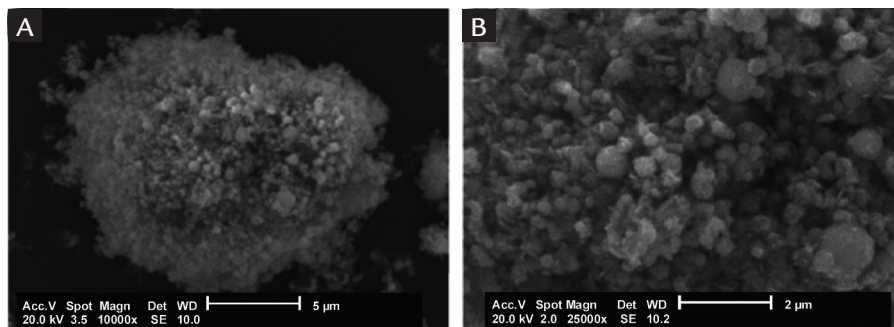
Figura 9 A) MEV's da lama fina de aciaria, mostrando a presença de aglomerados de partículas. B) Partículas com morfologia esférica.
