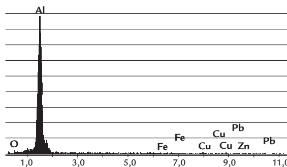
Figura 8 EDS da partícula mostrada na Figura 7B, indicando que tal partícula é, predominantemente, composta por alumínio, além de outros elementos em menor quantidade.
