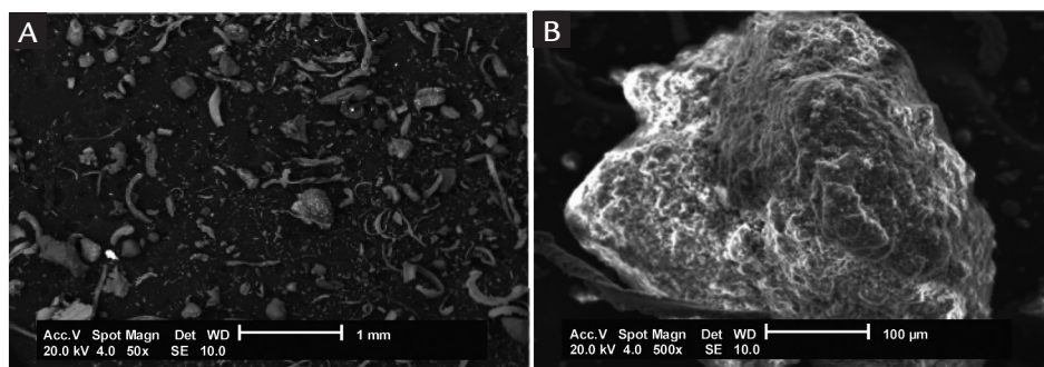
Figura 7 A) MEV's da borra de alumínio, mostrando partículas heterogêneas. B) Detalhe de uma típica partícula equiaxial.
