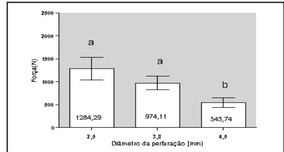
Figura 5- Média da força máxima de arrancamento dos parafusos de 5mm inseridos nos corpos das vértebras lombares de suínos e com diferentes diâmetros do orifício piloto.
