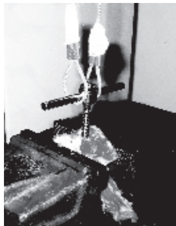
Figura 2 – Parafuso inserido na vértebra lombar de suíno e o dispositivo colocado na cabeça do parafuso para a aplicação da força durante o ensaio mecânico de arrancamento.
