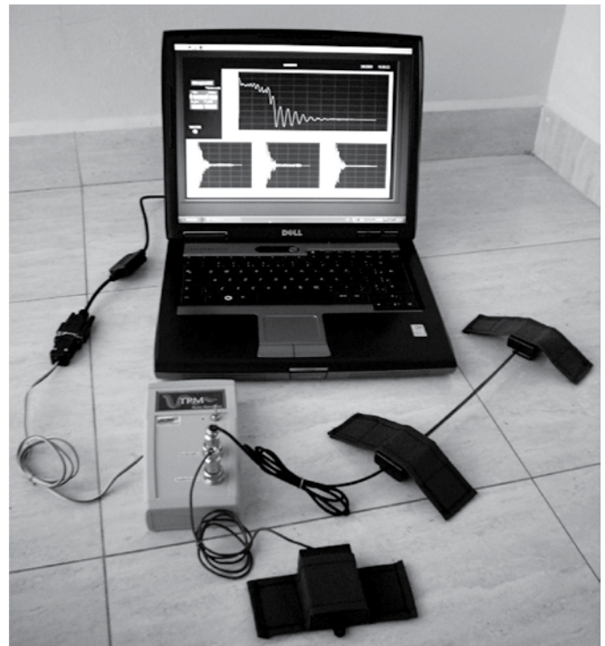
Figura 1. Equipamento DTP conectado ao computador.
