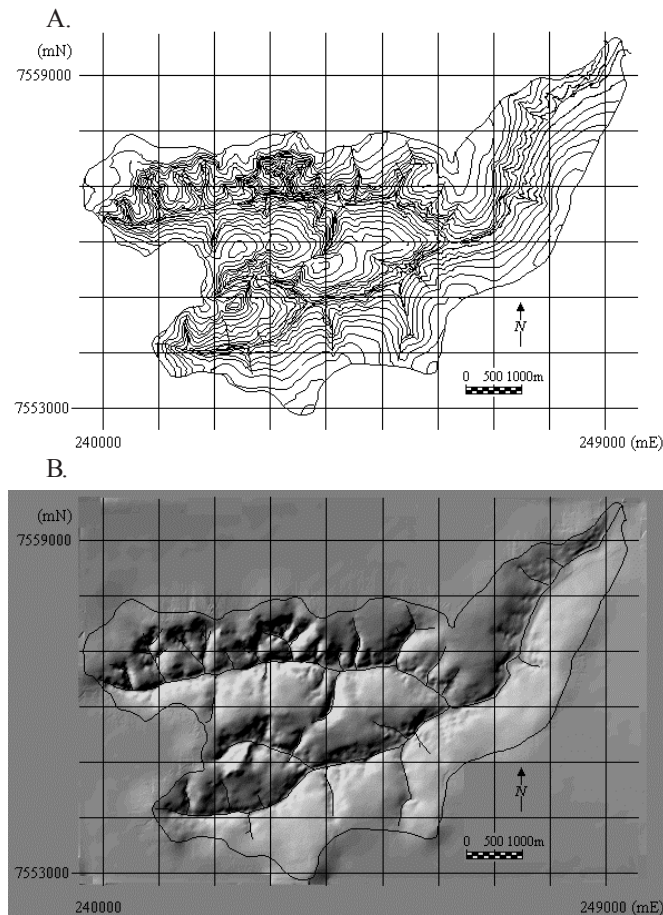
Figura 2. Curvas de nível digitalizadas (A) e o Modelo Digital de Terreno (MDT) formado com a resolução de 20 m (B)
