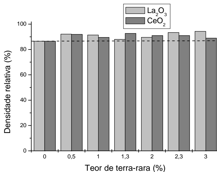
Figura 1: Densidade relativa das peças sinterizadas em 1400°C.
