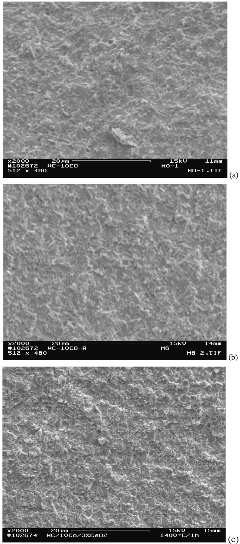
Figura 2: Micrografia das amostras WC/10Co sinterizadas (a) isenta de terra-rara (M0); (b) WC/10Co/3La 2 O 3 (M6); e (c) WC/10Co/3CeO 2 (M12).
