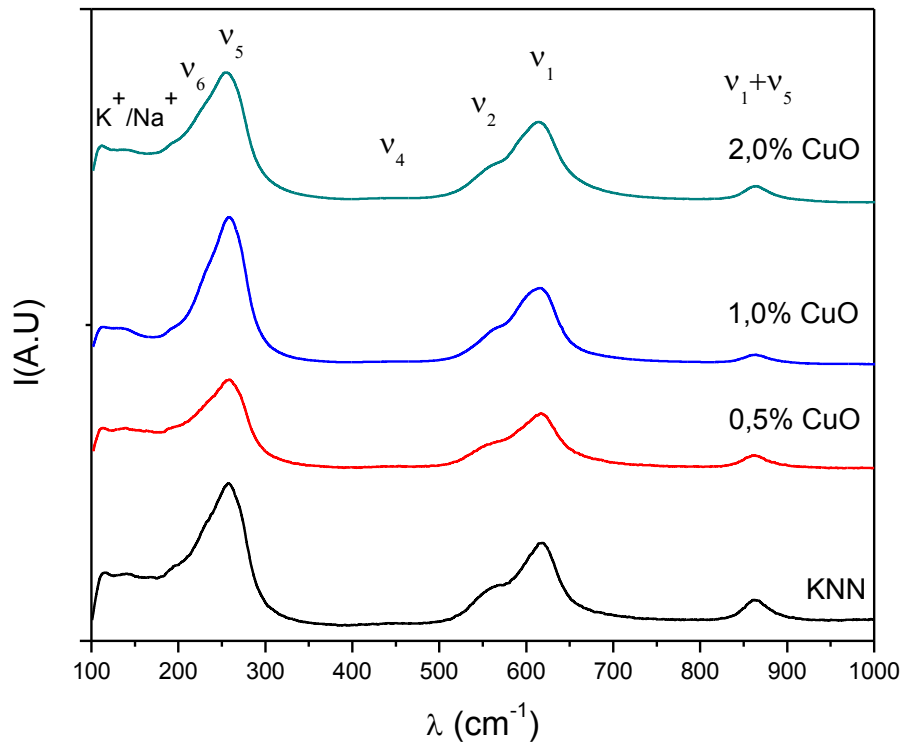
Figura 2. Espectro de Raman para KNN puro (0%) y KNN-dopado CuO como función de la concentración de aditivo (0 a 2% mol).
