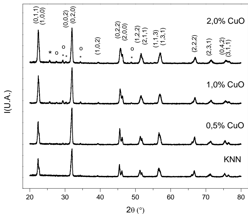
Figura 1. Patrón de DRX de KNN puro y KNN dopado con CuO. (*) Picos correspondientes a la fase K_2Nb_8O_{21} (JCPDS 26-13215) y (o) Picos correspondientes a la fase K_3NbO_4 (JCPDS 70-1148).
