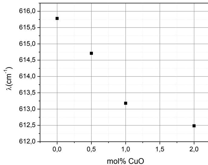
Figura 3. Longitud de onda de los modos de vibración A_{1g} ( v_1 ) en función de la concentración de CuO.
