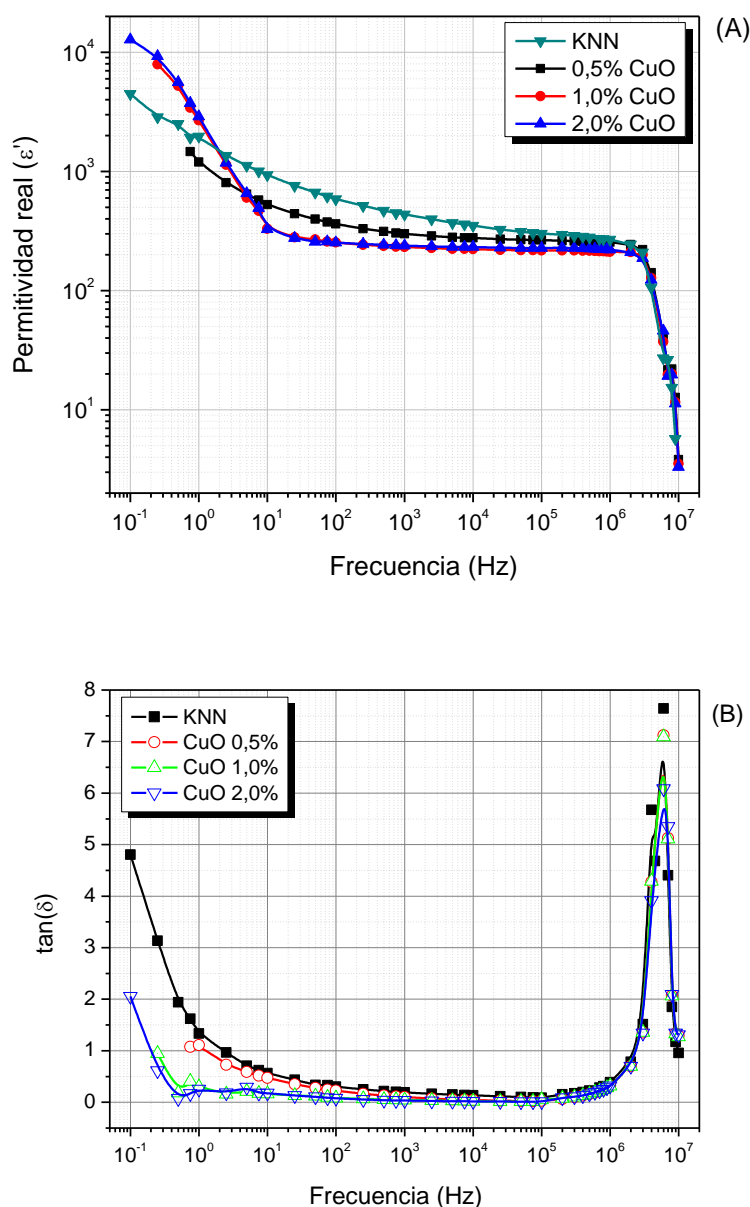
Figura 5. Variación de la permitividad real (A) y tangente de pérdida, \tan(\delta) , (B) como función de la frecuencia y la concentración de CuO, a temperatura ambiente.
