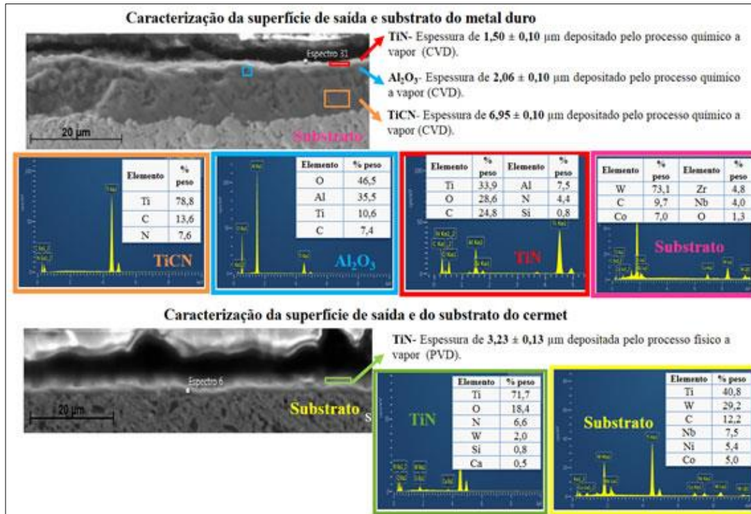
Figura 3: caracterização das camadas de revestimentos e substratos dos inserts de metal duro e cermet
