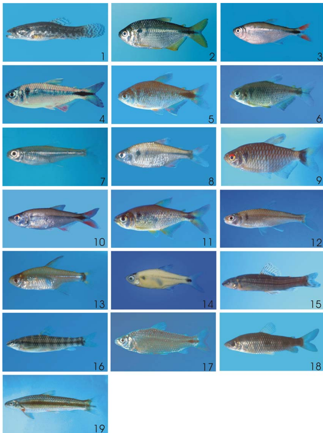
Figura 6. Exemplos representativos das espécies de peixes da ordem Characiformes coletadas na bacia do Rio Parapanema. Os respectivos números de registro na coleção ictiológica do LIRP e comprimentos padrões são apresentados após os nomes das espécies: 1) Hoplias malabaricus , LIRP 1694, 53,3 mm; 2) Astyanax altiparanae , LIRP 2878, 83,3 mm; 3) Astyanax fasciatus , LIRP 2755, 65,7 mm; 4) Astyanax scabripinnis , LIRP 2680, 61,3 mm; 5) Astyanax sp.1 , LIRP 2748, 48,2 mm; 6) Astyanax sp.2 , LIRP 2734, 94,6 mm; 7) Bryconamericus stramineus , LIRP 2793, 41,0 mm; 8) Bryconamericus sp. , LIRP 2784, 47,6 mm; 9) Moenkhausia sanctaefilomenae , LIRP 2390, 56,8 mm; 10) Oligosarcus paranaensis , LIRP 2395, 70,3 mm; 11) Oligosarcus pintoii , LIRP 1695, 52,0 mm; 12) Piabina argentea , LIRP 2418, 60,6 mm; 13) Serrapinnus notomelas , LIRP 2505, 24,5 mm; 14) Serrapinnus sp. , LIRP 2491, 25,0 mm; 15) Characidium gomesi , LIRP 2507, 56,1 mm; 16) Characidium zebra , LIRP 2518, 52,4 mm; 17) Cyphocharax modestus , LIRP 2347, 104,1 mm; 18) Leporinus paranensis , LIRP 2254, 101,5 mm; 19) Apareiodon piracicabae , LIRP 2553, 90,8 mm (Fotos Alexandre C. Ribeiro, Alex L. A. Melo e Ricardo M. C. Castro).
