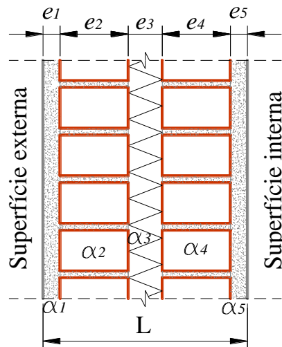
Figura 3 - Detalhe da parede composta por materiais de difusividades térmicas \alpha_1, \alpha_2, \dots, \alpha_5 e espessuras e_1, e_2, \dots, e_5
