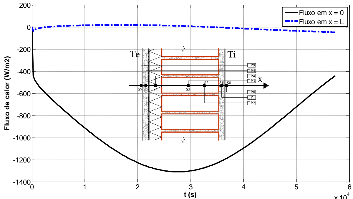
Figura 6 - Fluxo de calor na Parede 4
