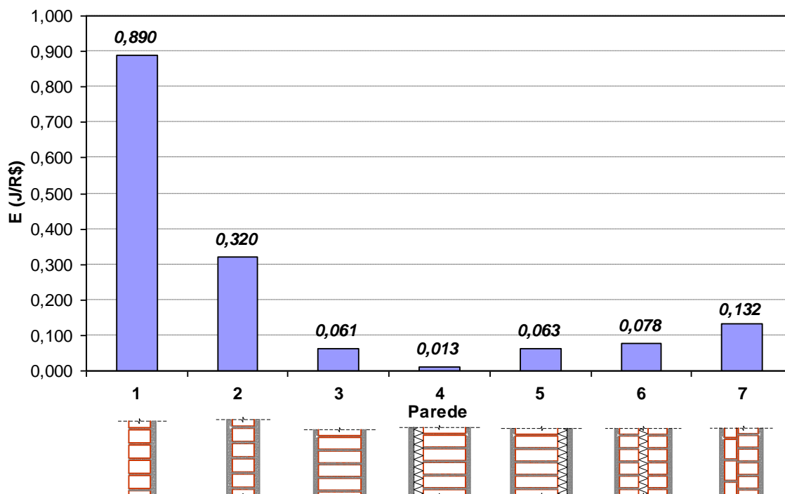
Figura 8 - Relação termoeconômica das paredes
