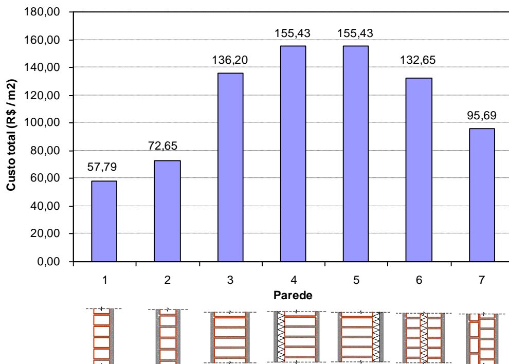
Figura 7 - Custo total por metro quadrado das paredes estudadas
