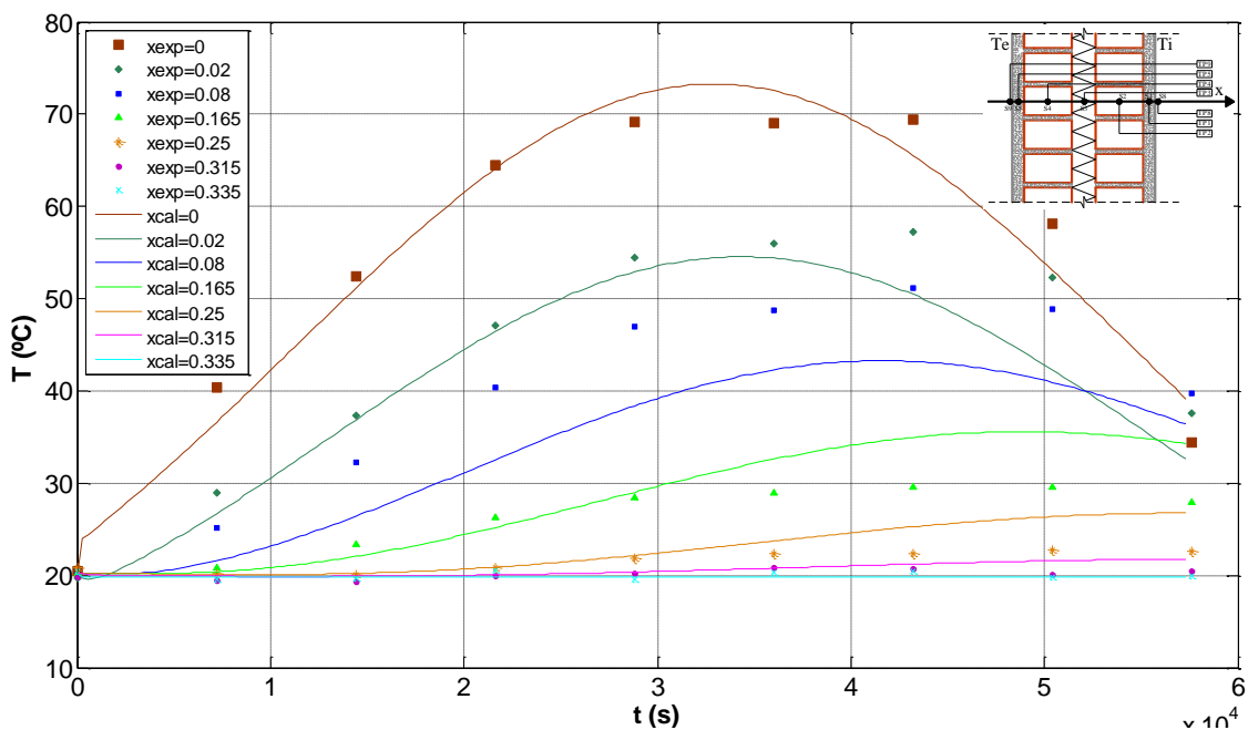
Figura 5 - Comparação dos dados experimentais com os resultados calculados com as difusividades da Tabela 1 para a Parede 6
