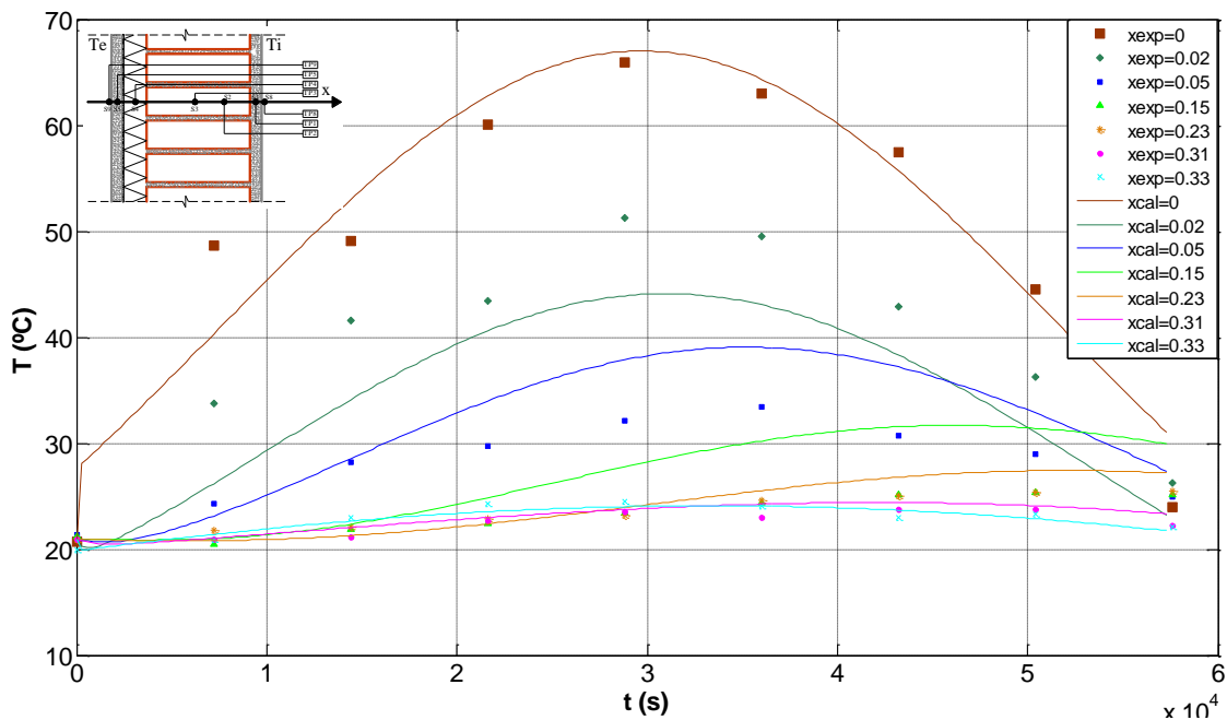
Figura 4 - Comparação dos dados experimentais com os resultados calculados com as difusividades da Tabela 1 para a Parede 4
