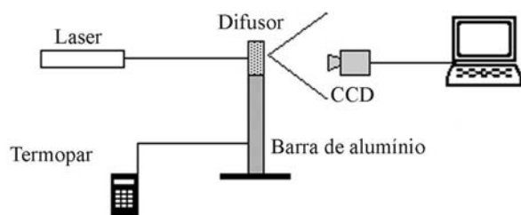
Figura 5 - Arranjo experimental.
