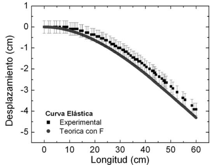
Figura 10 - Curva elástica de la lámina sometida a una fuerza de 4,214 N en el extremo libre, un módulo de Young de 66 GPa (calculado para un vidrio en un ensayo destructivo). Ancho del vidrio 2 cm, espesor 0.4 cm, longitud 60 cm y peso del vidrio 127,2 g.
