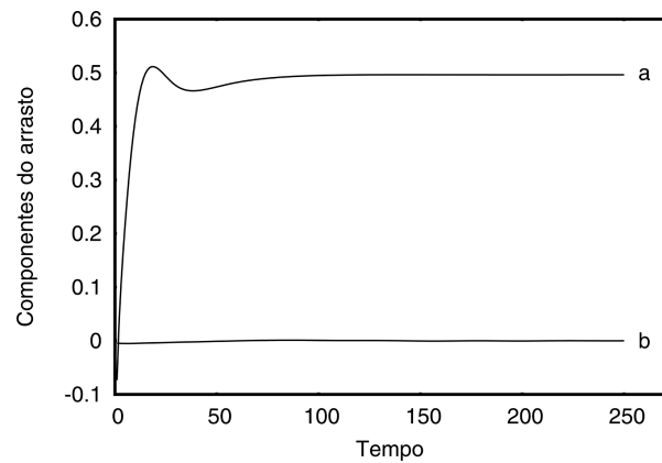
Figura 4: Componentes do arrasto para ângulo de ataque igual a 0^\circ . Em (a), apresenta-se a componente longitudinal e, em (b), a componente transversal. A componente longitudinal cresce, atinge um valor máximo, reduz-se um pouco e se estabiliza, passando a oscilar levemente (imperceptível na figura) em torno de um valor fixo positivo, enquanto a componente transversal, após o transiente, passa a flutuar em torno de um valor fixo, no caso do ângulo de ataque igual a 0^\circ , este valor é nulo, como esperado para obstáculos simétricos.
