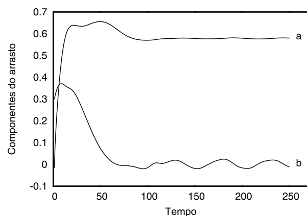
Figura 5: Componentes do arrasto para ângulo de ataque igual a 15^\circ . Em (a), apresenta-se a componente longitudinal e, em (b), a componente transversal. Assim como antes, a componente longitudinal cresce, atinge um valor máximo, reduz-se um pouco e estabiliza, passando a oscilar em torno de um valor fixo positivo enquanto a componente transversal, após o transiente (neste caso, bem diferente do caso para ângulo de ataque 0^\circ , pois a simetria axial foi quebrada), passa a flutuar em torno de um valor fixo, no caso do ângulo de ataque igual a 15^\circ , este valor é positivo, embora pequeno se comparado com a componente longitudinal.
