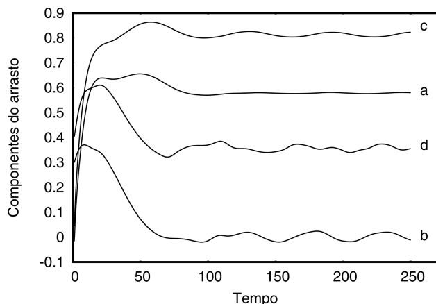
Figura 7: Comparação das componentes do arrasto para a asa com e sem flap para um ângulo de ataque igual 15^\circ . Em (a) e (b), se observam, respectivamente, as componentes longitudinal e transversal do arrasto para asa sem flap (repetido da Fig. 5) enquanto em (c) e (d), se observam, respectivamente, as componentes longitudinal e transversal do arrasto para asa com flap. Como esperado, para um mesmo ângulo de ataque, a asa com flap apresenta valores mais altos para suas componentes embora o comportamento qualitativo seja aproximadamente o mesmo com ou sem flap.
