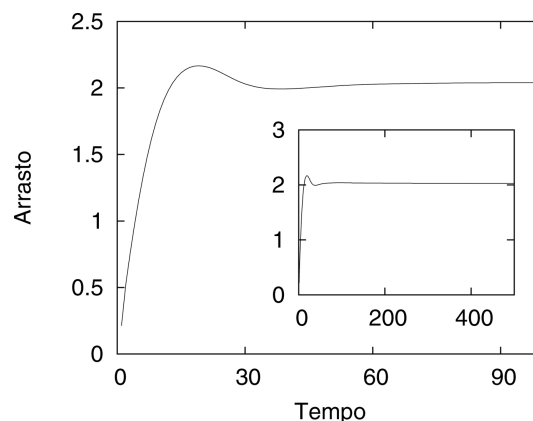
Figura 2: Força de arrasto sobre um cilindro estático no túnel de vento. Inicialmente o túnel está desligado. Em seguida, em t = 0 , o túnel é ligado com número de Reynolds Re = 1000 . A componente da força na direção perpendicular ao fluxo do vento é desprezível. A força de arrasto é representada em unidades arbitrárias, ignorando fatores como a densidade do fluido, etc. Durante uma unidade de tempo, o vento viaja o equivalente ao diâmetro do cilindro. A componente da força que é paralela ao fluxo de vento aumenta, atinge um valor máximo, diminui e finalmente se estabiliza, o que corresponde a uma situação dinâmica em que aparecem continuamente vórtices sucessivos girando em sentidos alternados atrás do cilindro. A esteira de vórtices de von Kármán é então formada. O destaque mostra o mesmo numa escala longa no tempo.
