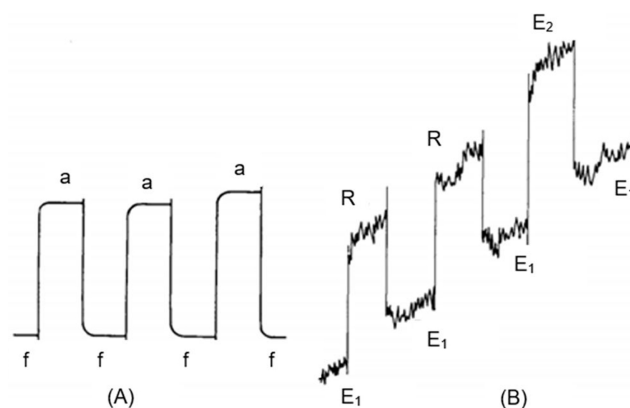
Figura 4: Saída do detector com o obturador aberto (a) e fechado (f) de um radiômetro absoluto (A) e diferencial ( offset ) em resposta ao aquecimento devido a uma potência elétrica de valor conhecido ( E_1 ) e a potência radiante desconhecida (R), adaptado de [22].
