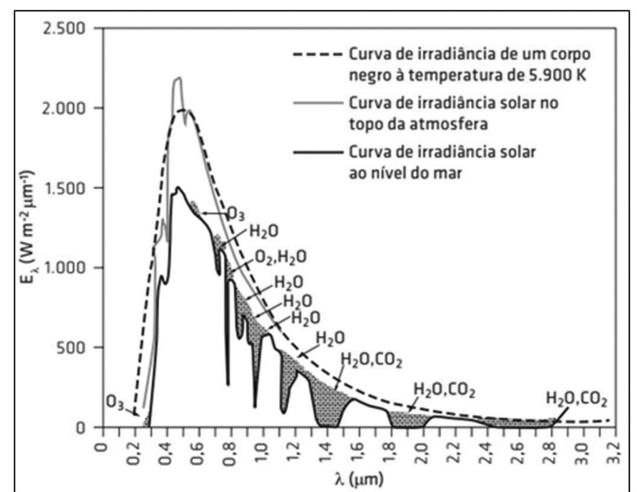
Figura 2: Intensidade do fluxo radiante emitido pelo Sol. Comparação do espectro solar medido fora da atmosfera terrestre, irradiância solar padrão ao nível do mar, espectro de um corpo negro a 5.900K e identificação de regiões espectrais que ocorrem absorção molecular [7].
