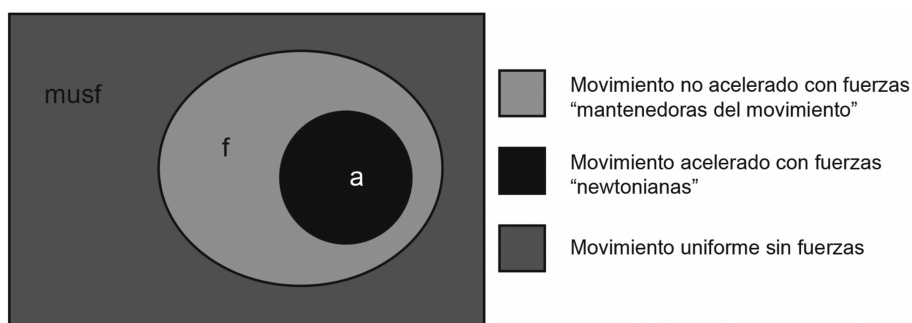
Figura 2: 1ª Ley de Newton a \rightarrow f
