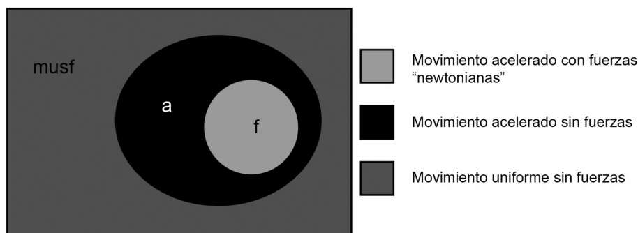
Figura 3: Definición de fuerza newtoniana f \rightarrow a
