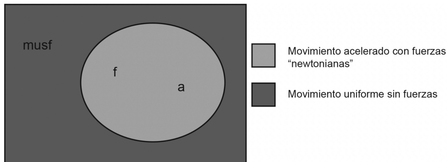
Figura 4: Relación entre fuerza y aceleración, aceptada actualmente por los científicos. a \leftrightarrow f
