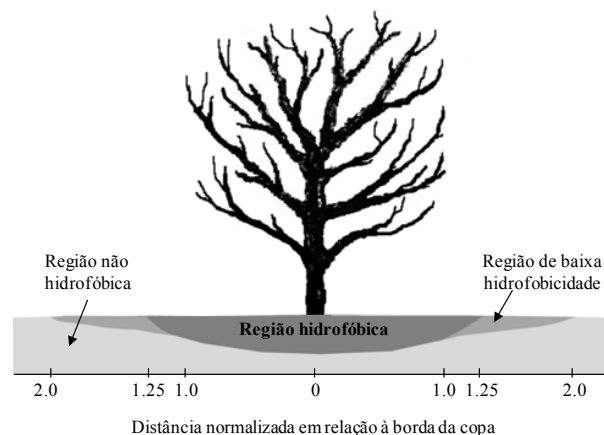
FIGURA 2: Diagrama esquemático do dossel de uma árvore após ocorrência de um incêndio, evidenciando as áreas hidrofóbicas, de baixa hidrofobicidade e não hidrofóbicas (Adaptado de: Madsen et al., 2011; reproduzido/adaptado com permissão de Soil Science Society of American Journal).
