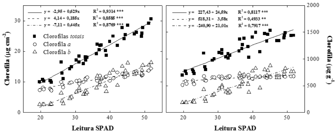
FIGURA 1: Relação entre valores de leitura SPAD e teores (expressos em \mu\text{g cm}^{-2} e \mu\text{g g}^{-1} ) de clorofilas ( totais , a e b ) em folhas de vime ( Salix viminalis ). ** e *** para níveis de significância, nos modelos ajustados, de 0,01 e 0,001, respectivamente.
